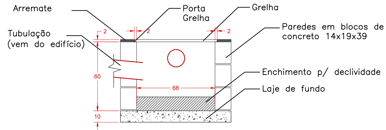
CANALETA EM CORTE ESC. 1 :20
