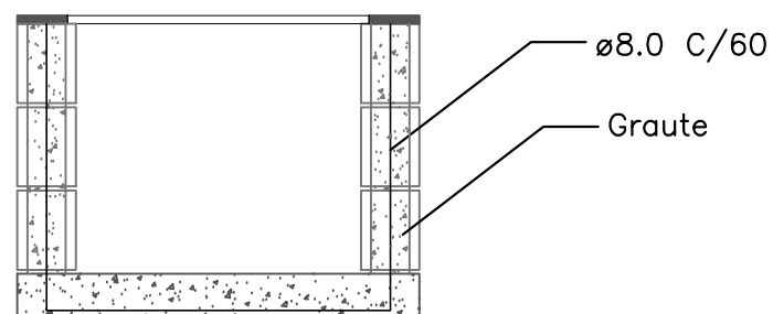
DETALHE ARMADURA CANALETA ESC. 1 :20
